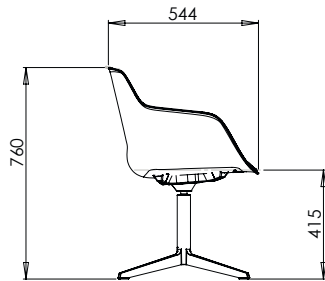
FourMe Lounge, Rembourrage de la face intérieure
