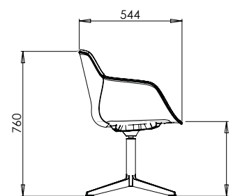
FourMe Lounge, Rembourrage intégral
