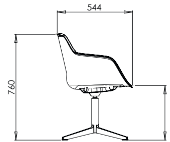
FourMe Lounge, Rembourrage de l'assise
